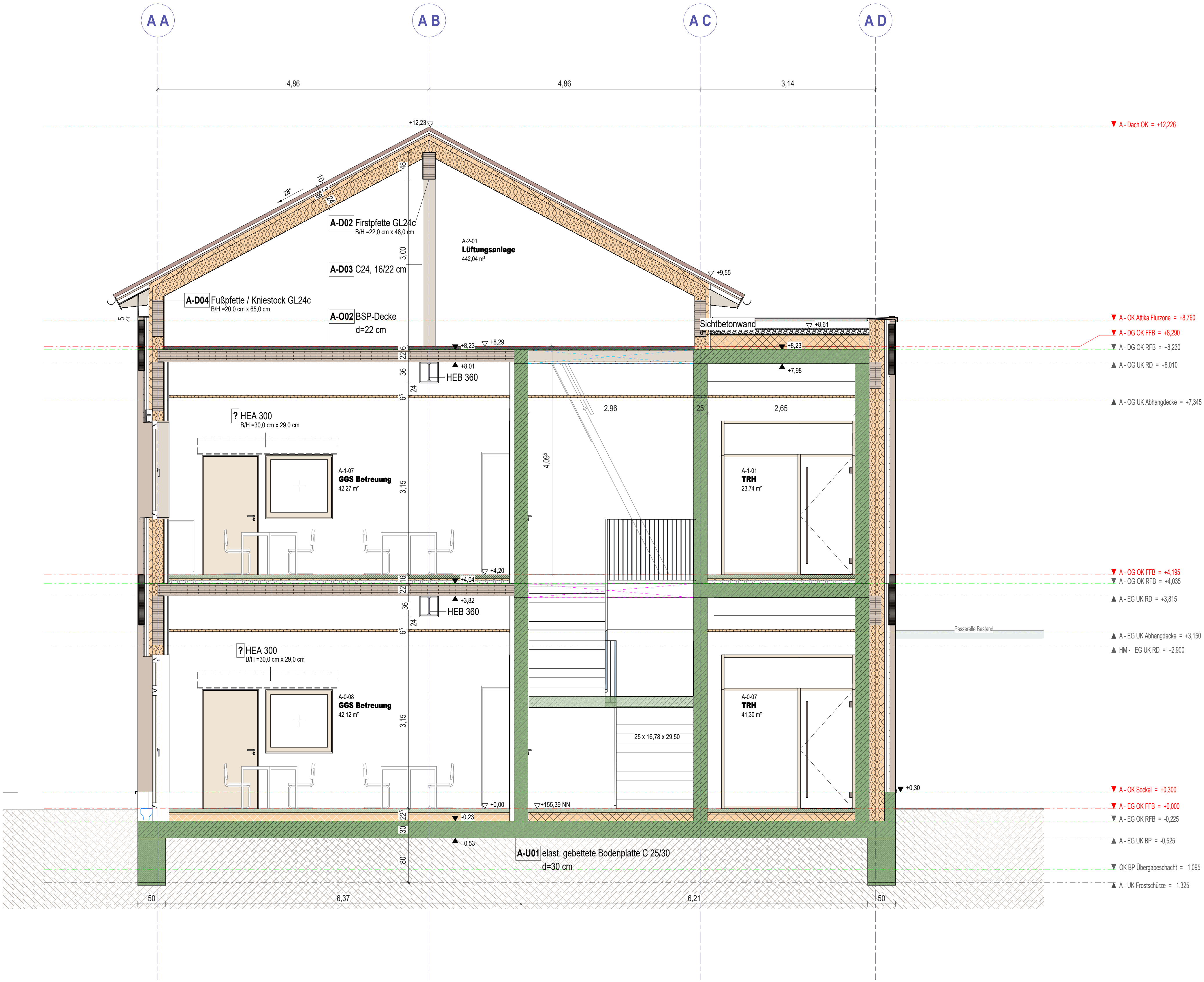
Schnitt A1 M 1 : 50
