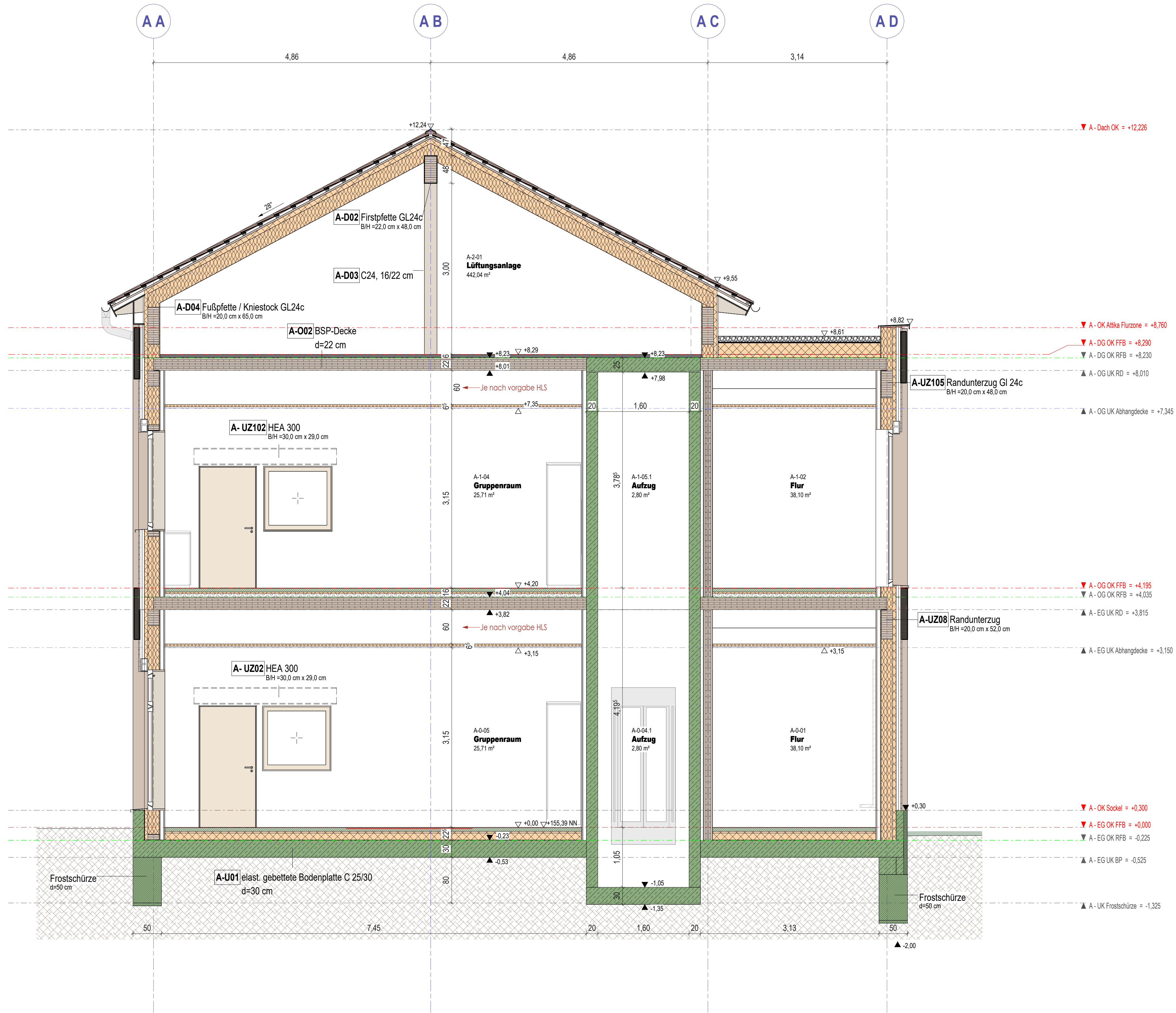
Schnitt A2 M 1 : 50
